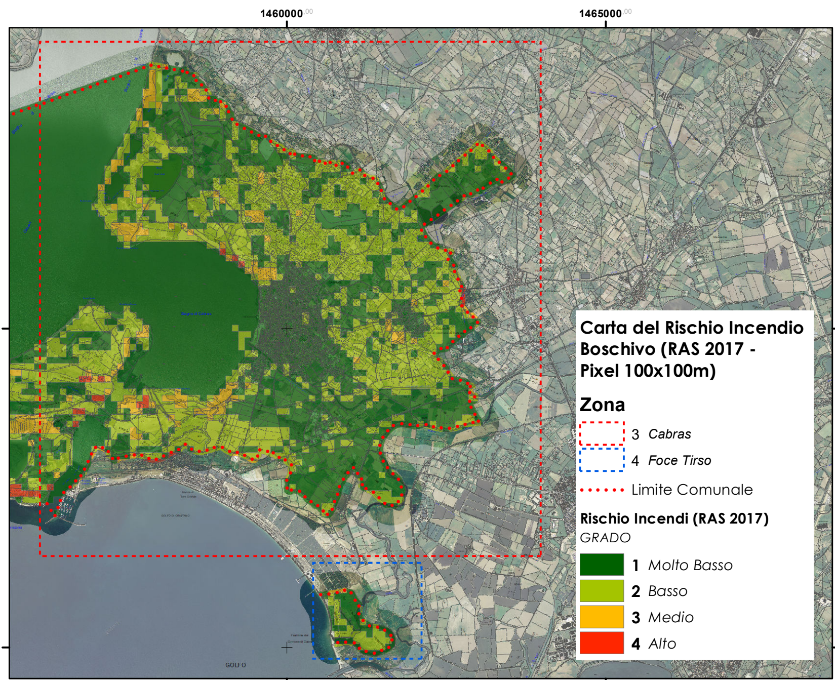
Carta del Rischio Incendio Boschivo (RAS 2017) Sc.1:60.000
