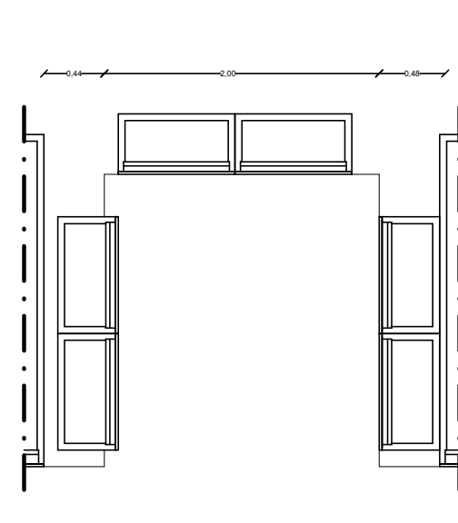
pianta 1:50
