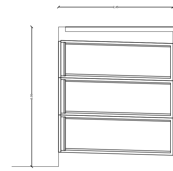
sezione 1:50
