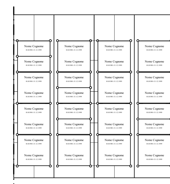
prospetto frontale 1:50
